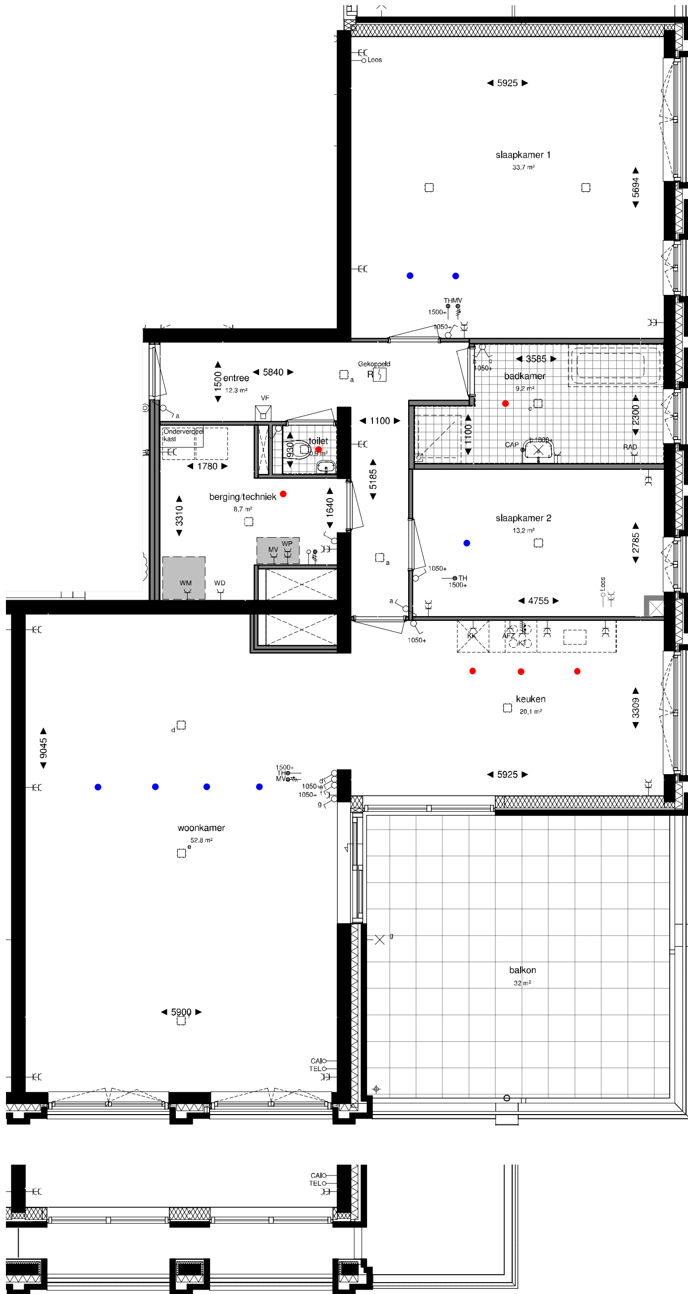
Gevelindeling type 08, 6e verdieping
